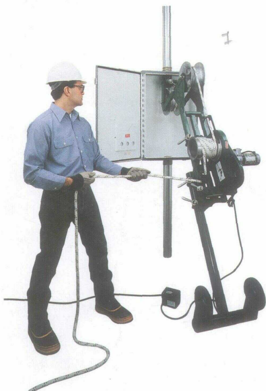
Optional Force Gauge
