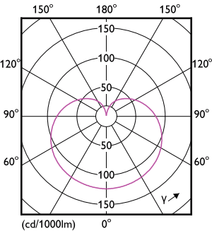
Light Distribution Diagram - 8.8A19/MAS/927-22/FR/P/E26/T20 6/1CT
