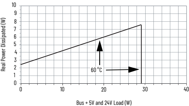
1769-PB2, 1769-PB2K Power Dissipation
