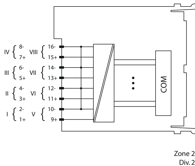
I/O Module
