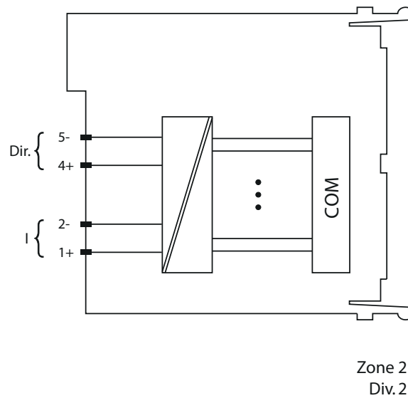
I/O Module
