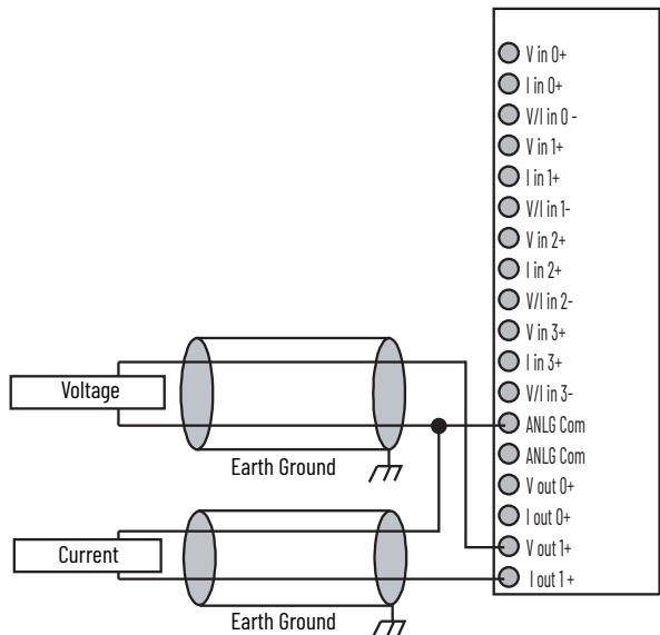
Analogue Output Wiring
