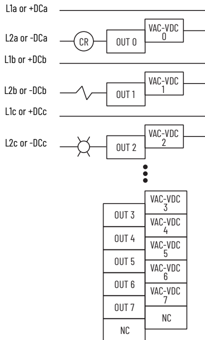
Output Wiring
