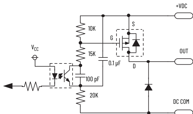
Output Wiring
