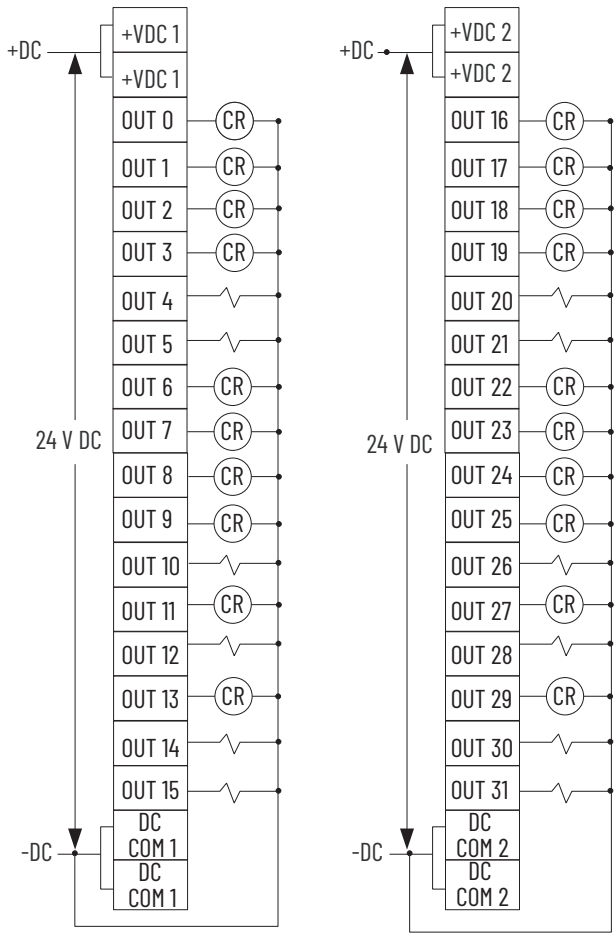
Output Wiring
