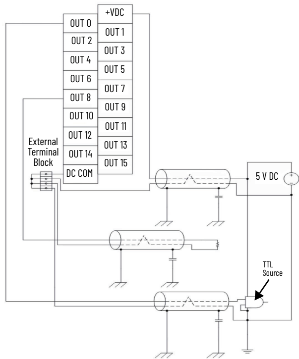
Output Wiring
