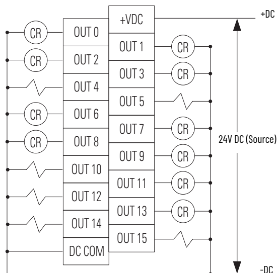
Output Wiring
