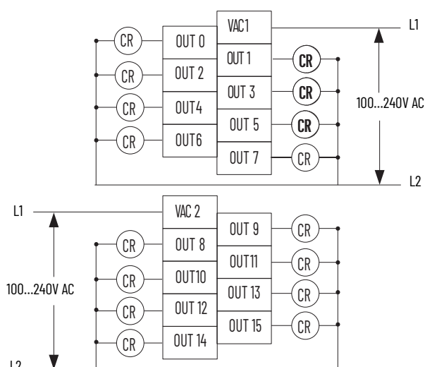
Output Wiring
