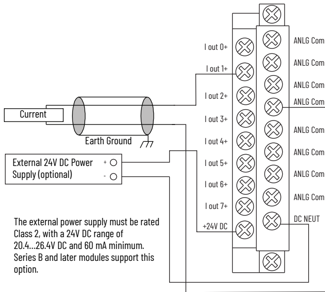
Output Wiring
